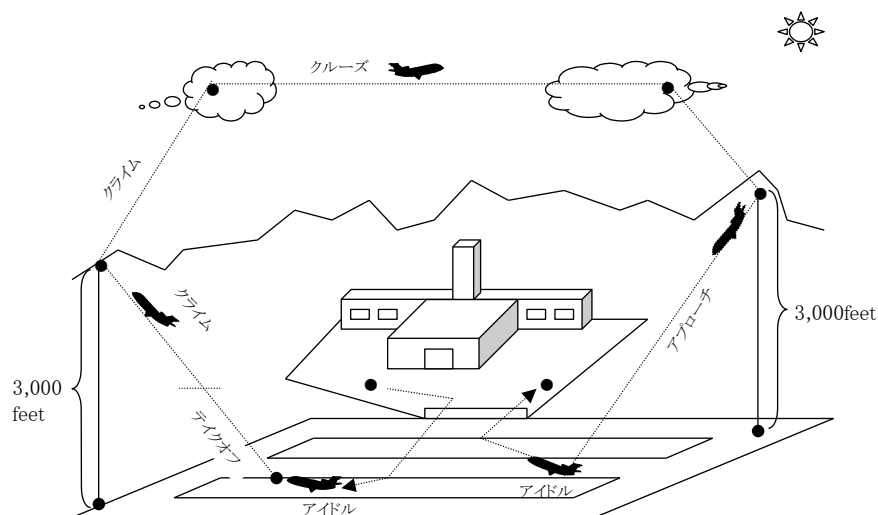
図 16-1 航空機に係る LTO サイクル
