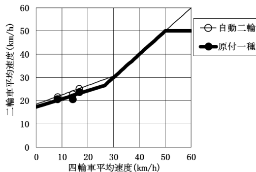
図12-1 四輪車の速度と二輪車の速度の関係
