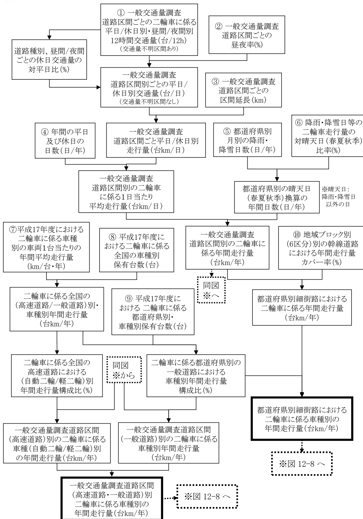
図12-7 一般交通量調査道路区間別及び細街路年間走行量の推計フロー
