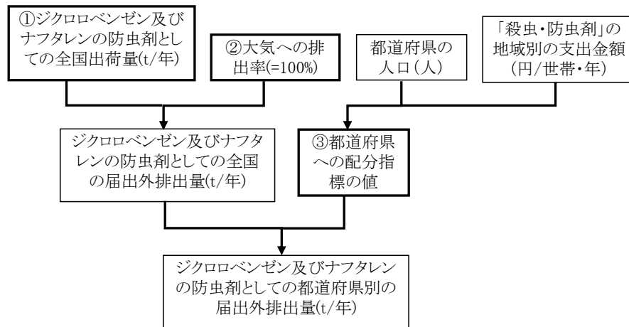
図 8-1 防虫剤に係る排出量の推計フロー
