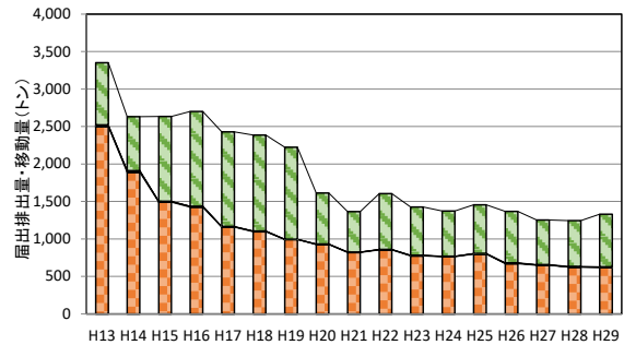
ベンゼン(400)
