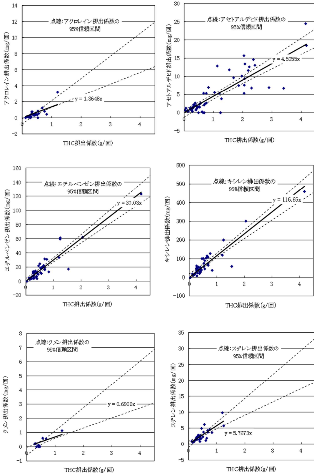
出典:環境省環境管理技術室(平成14年) 図 11-43 ガソリン自動車(コールドスタート時の増分)に係る THC 排出量と対象化学物質別排出量の比率(その1)
