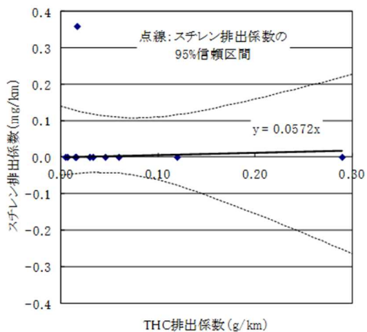
図 11-40 ディーゼル自動車(ホットスタート:重量車以外(触媒あり))に係る THC 排出量と対象化学物質別排出量の比率(その1)
