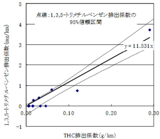
図 11-40 ディーゼル自動車(ホットスタート:重量車以外(触媒あり))に係る THC 排出量と対象化学物質別排出量の比率(その1)
