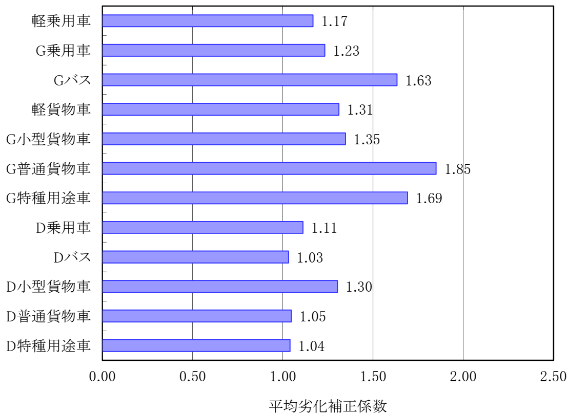
図 11-13 平均劣化補正係数の推計結果(平成 30 年度)
