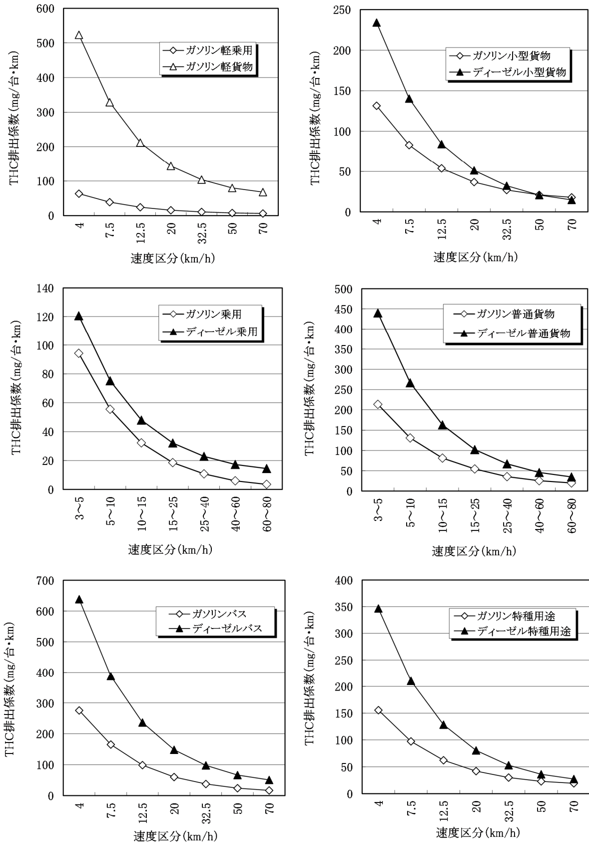
図 11-14 車種別・旅行速度区別の THC 排出係数(平成 30 年度:触媒の劣化補正後)
