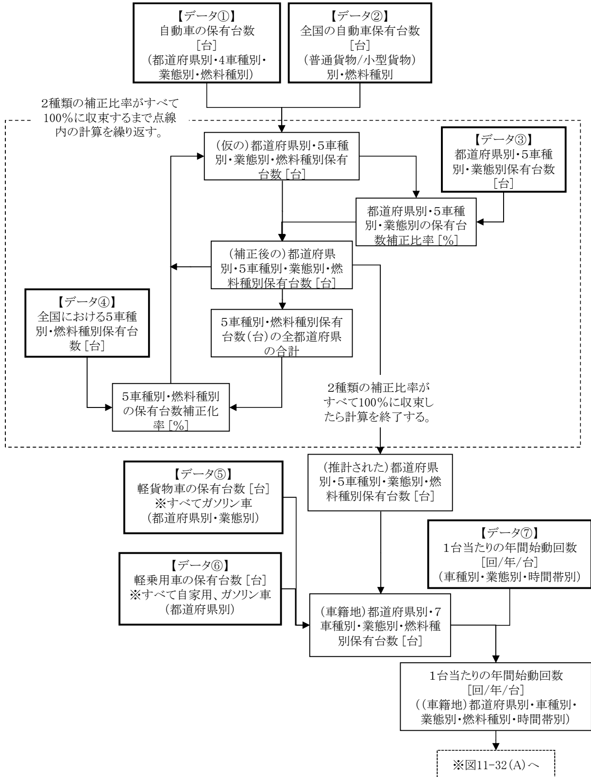
図 11-30 都道府県別・車種別・業態別・燃料別・時間帯別始動回数の推計フロー
