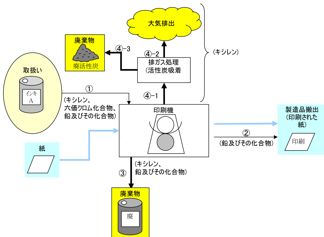
図 1-6-1 印刷施設(1)の概要図
