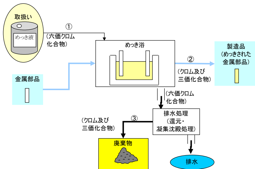
図 1-8-2 めっき施設(2)の概要図
