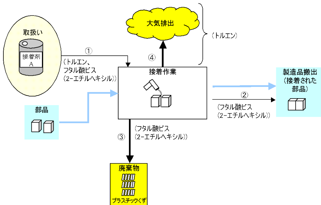
図 1-7-1 接着施設(1)の概要図
