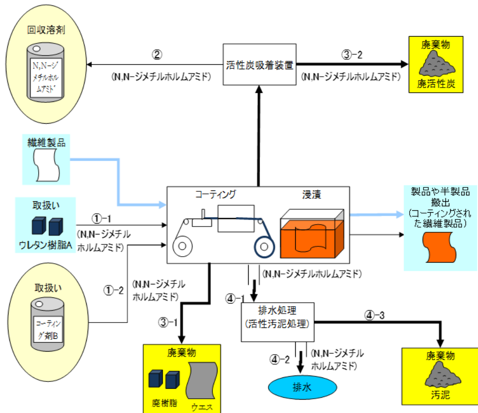
図 1-9-2 コーティング施設(1)の概要図
