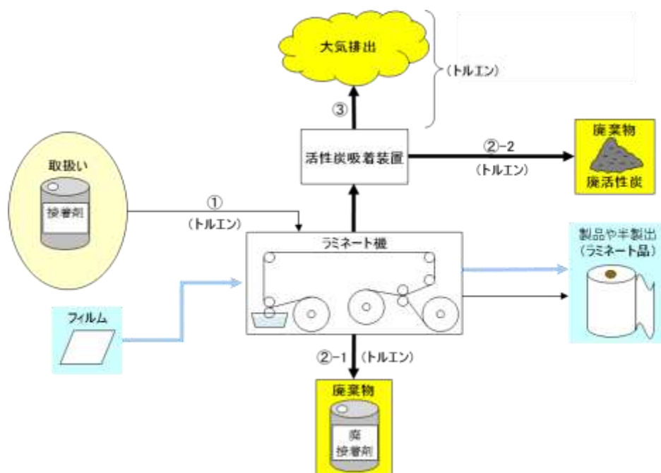
図 1-7-2 ラミネート施設の概要図
