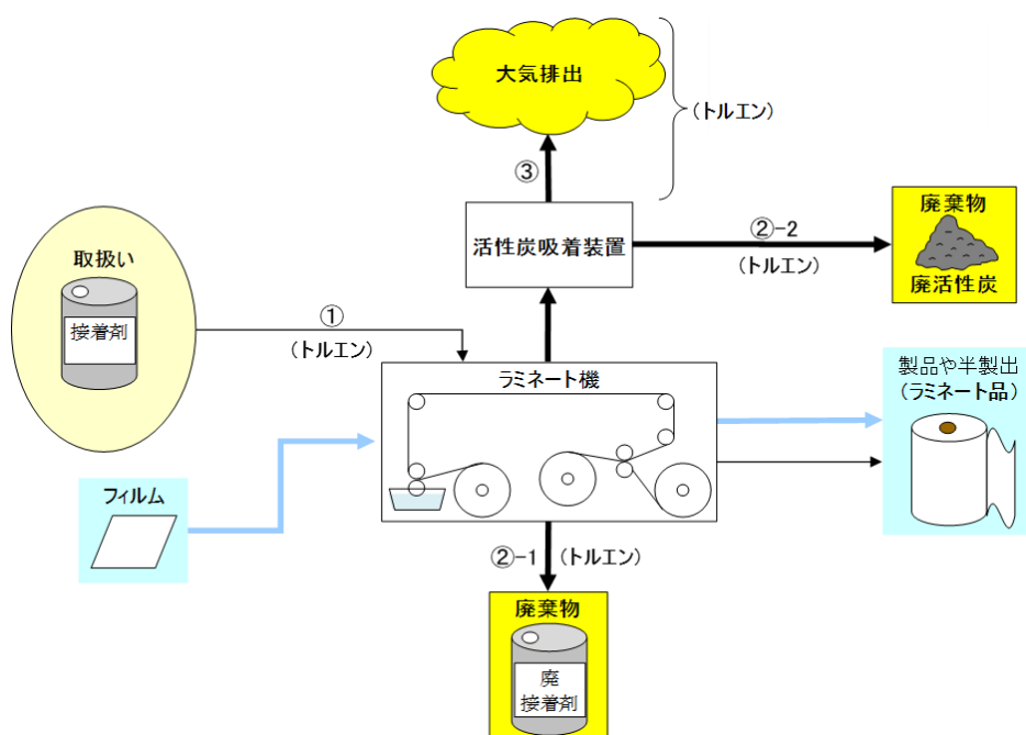
図 1-7-2 ラミネート施設の概要図
