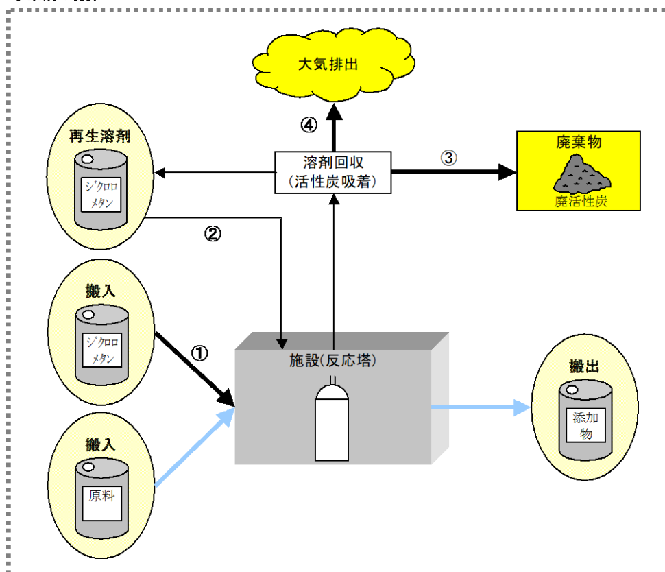
図 1-2-4 反応施設(4)の概要図
