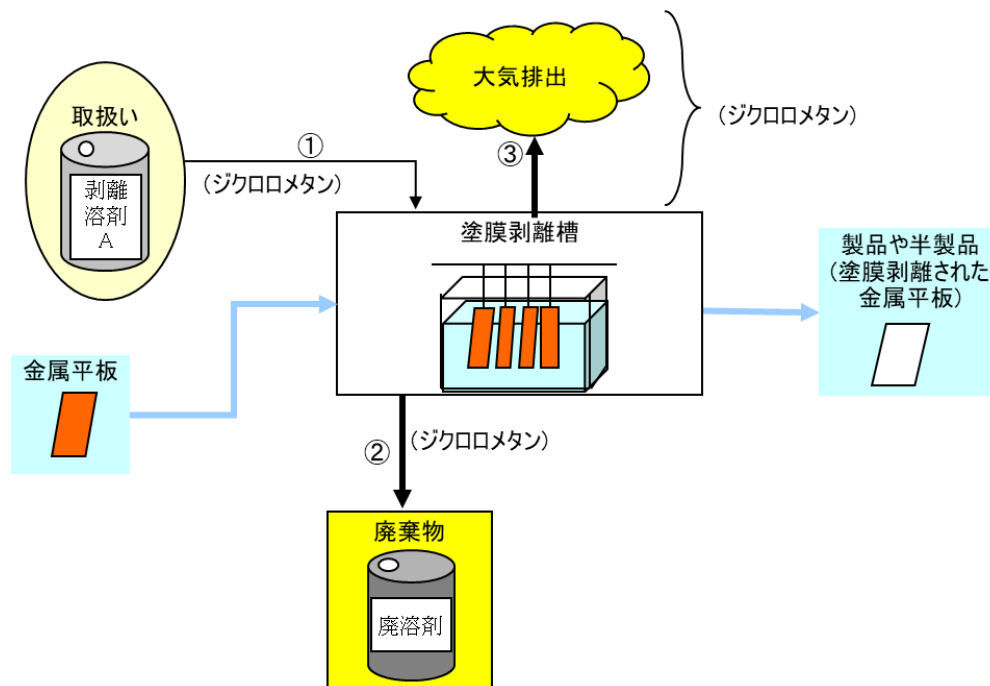
図 1-11 剥離施設の概要図
