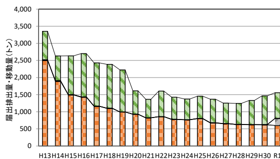
ベンゼン(400)
