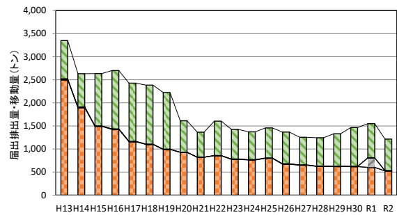
ベンゼン(400)
