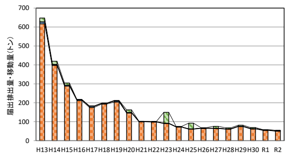
1,3-ブタジエン(351)
