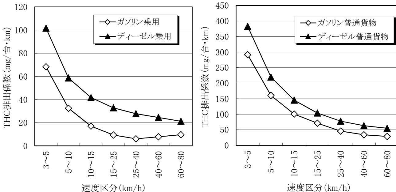
図1 車種別・速度区別の THC 排出係数の例 (令和2年度)
