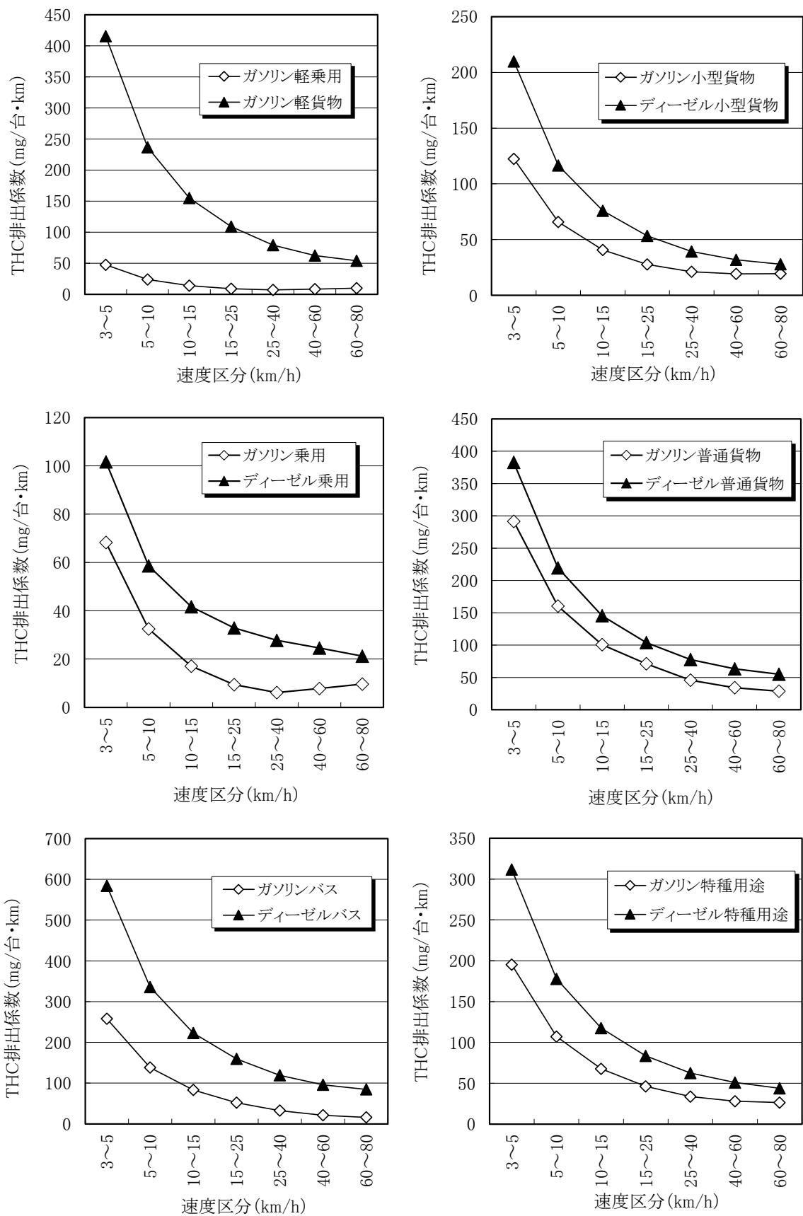
図 11-14 車種別・旅行速度区分別の THC 排出係数(令和2年度:触媒の劣化補正後)
