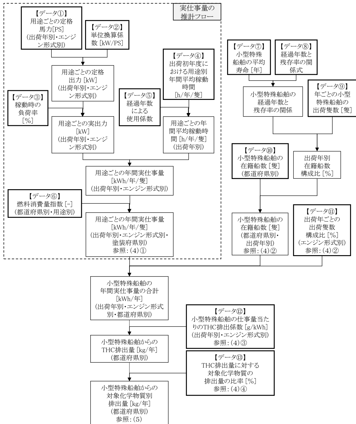
図 14-10 特殊小型船舶に係る対象化学物質別排出量の推計フロー
