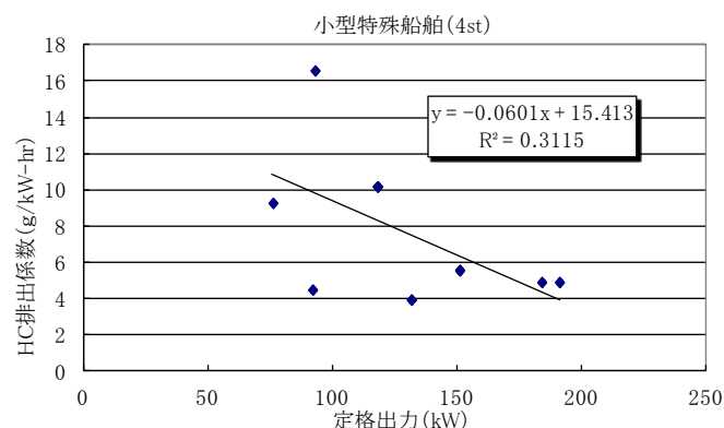
図 14-14 定格出力と THC 排出係数の関係の例(特殊小型船舶(4ストローク))
