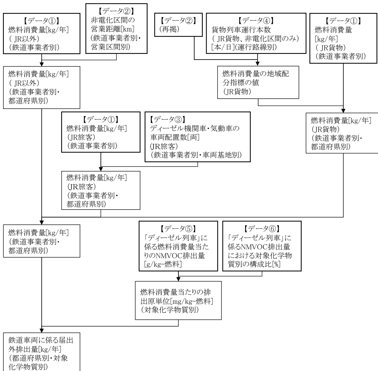
図 0-1 鉄道車両(エンジン)に係る排出量の推計フロー
