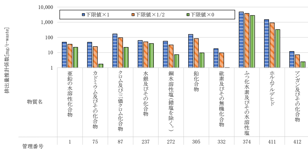
図 22-4 焼却施設の排ガスに係る焼却処理量1トン当たりの化学物質排出量
