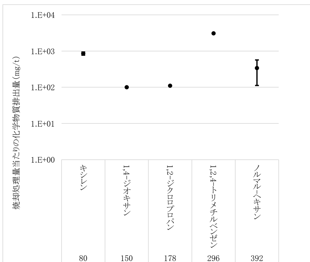
図 23-7 焼却処理量1トン当たりの化学物質排出量(有機化合物)
