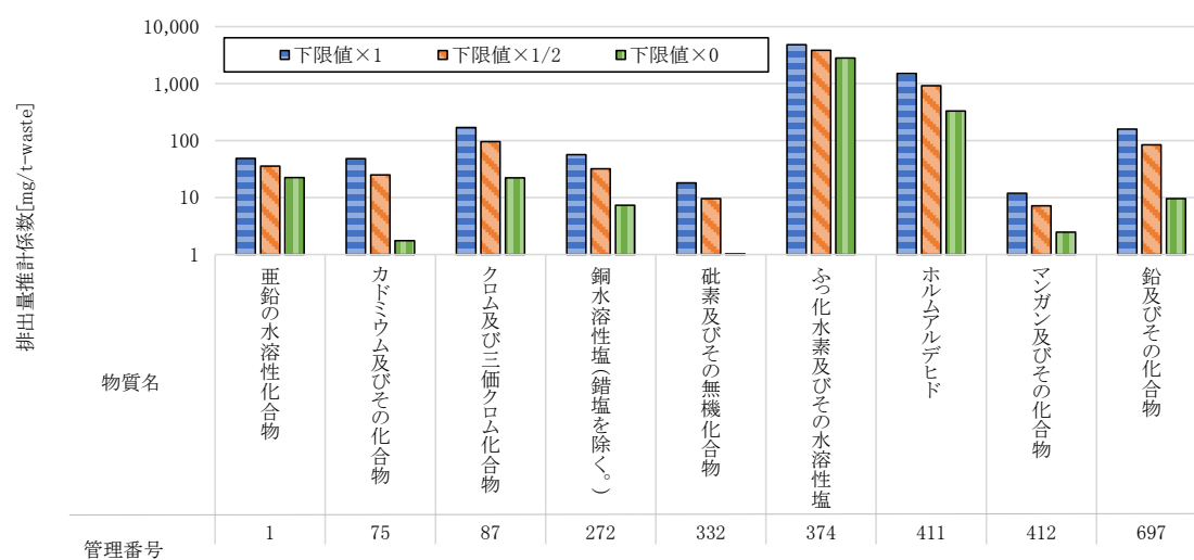
図 22-4 焼却施設の排ガスに係る焼却処理量 1 トン当たりの化学物質排出量
