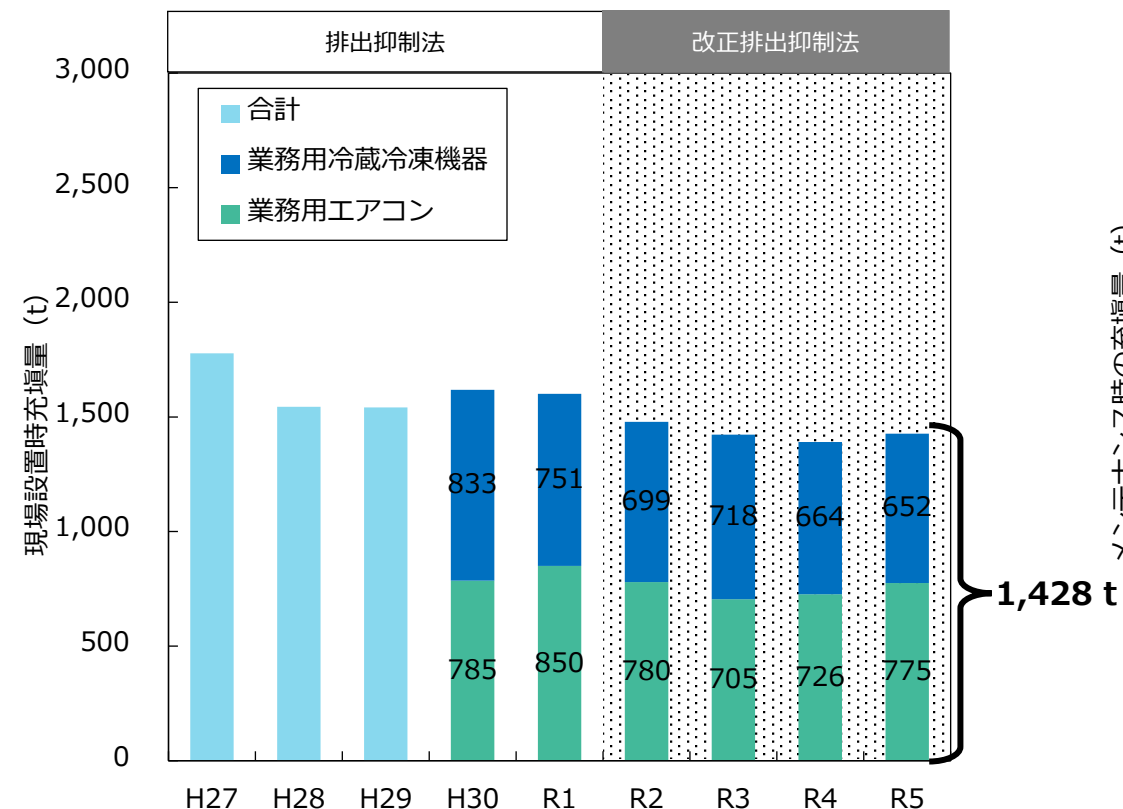
新設機器の現場設置時の充填量 (HFCsのみ)
