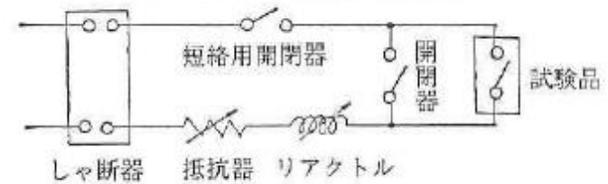
図1 单相2線式で単極の場合
