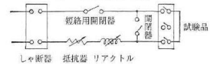
図3 单相3線式の場合
