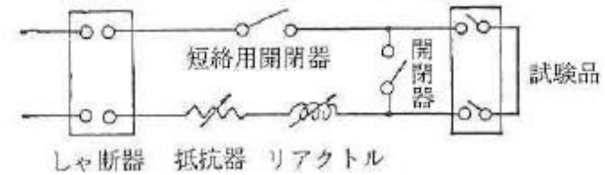
図2 单相2線式で2極の場合
