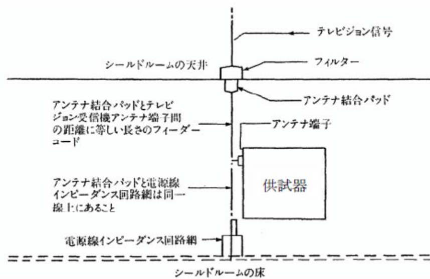
図 3-15 供試品の配置
