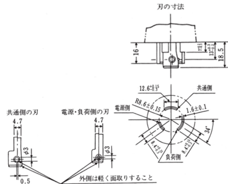
図1 本体（刃側）の接続部寸法
