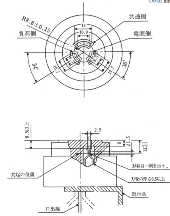
図2 受台（刃受側）の接続部寸法
