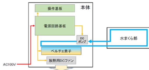
ブロック図
