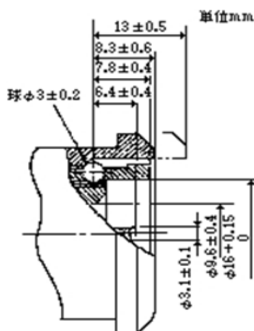
図1 ソケット
