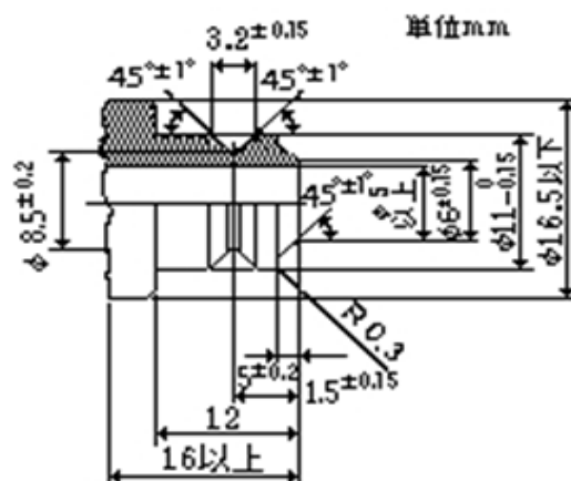
図 2 プラグ
