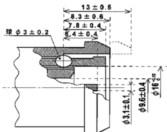
図２ プラグ 単位mm
