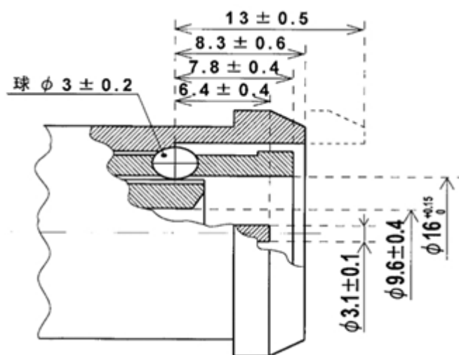
図1 ソケット 単位mm
