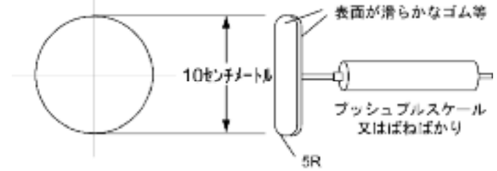
図 3-2 円板当て板
