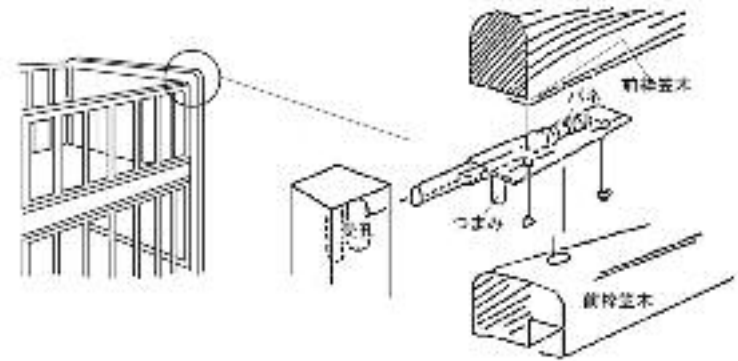
図 3 - 1 - 3
