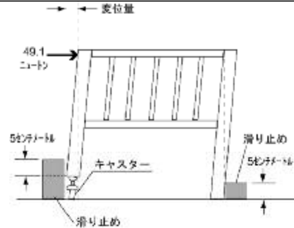
図 3 - 9 - 2
