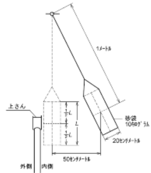
図 3 - 1 0
