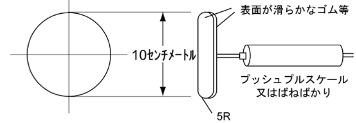
図 3 - 2 円板当て板
