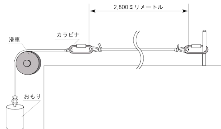
図4-2 有効長測定点
