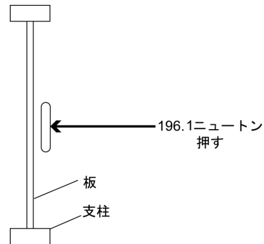
図 3-8-2 板の場合
