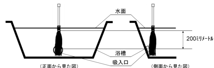
図6-4 試験用毛髪を吸入口に置く例
