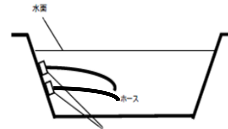
ジェット噴出口と吸入口
