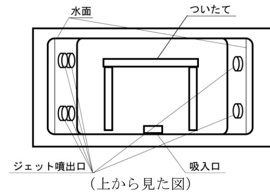
図6-5-1 ジェット噴流機能等の影響を少なくさせる措置の例（ついたてを用いたもの）
