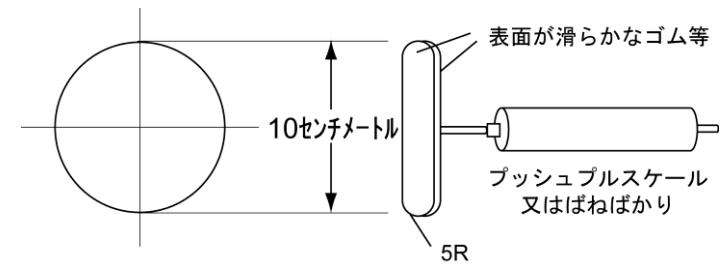
図 3 - 2 円板当て板
