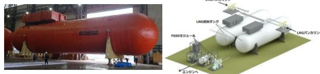
現在のLNG燃料タンク、燃料供給システム
