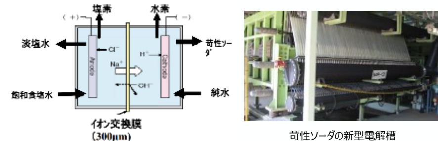
＜電解装置（イオン交換膜法）＞
