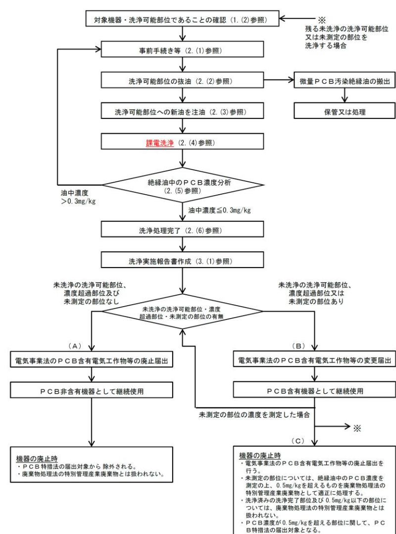
図1 課電洗浄フロー図
