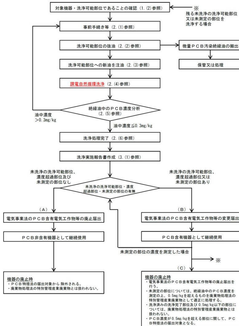
図1 課電自然循環洗浄フロー図
