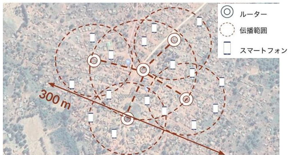
メッシュネットワークの村への設置 イメージ図
