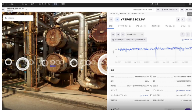
（図2）装置の3D画像と関連データを同時表示
