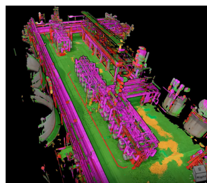
（図3）AIにより装置を自動認識・識別した画像
