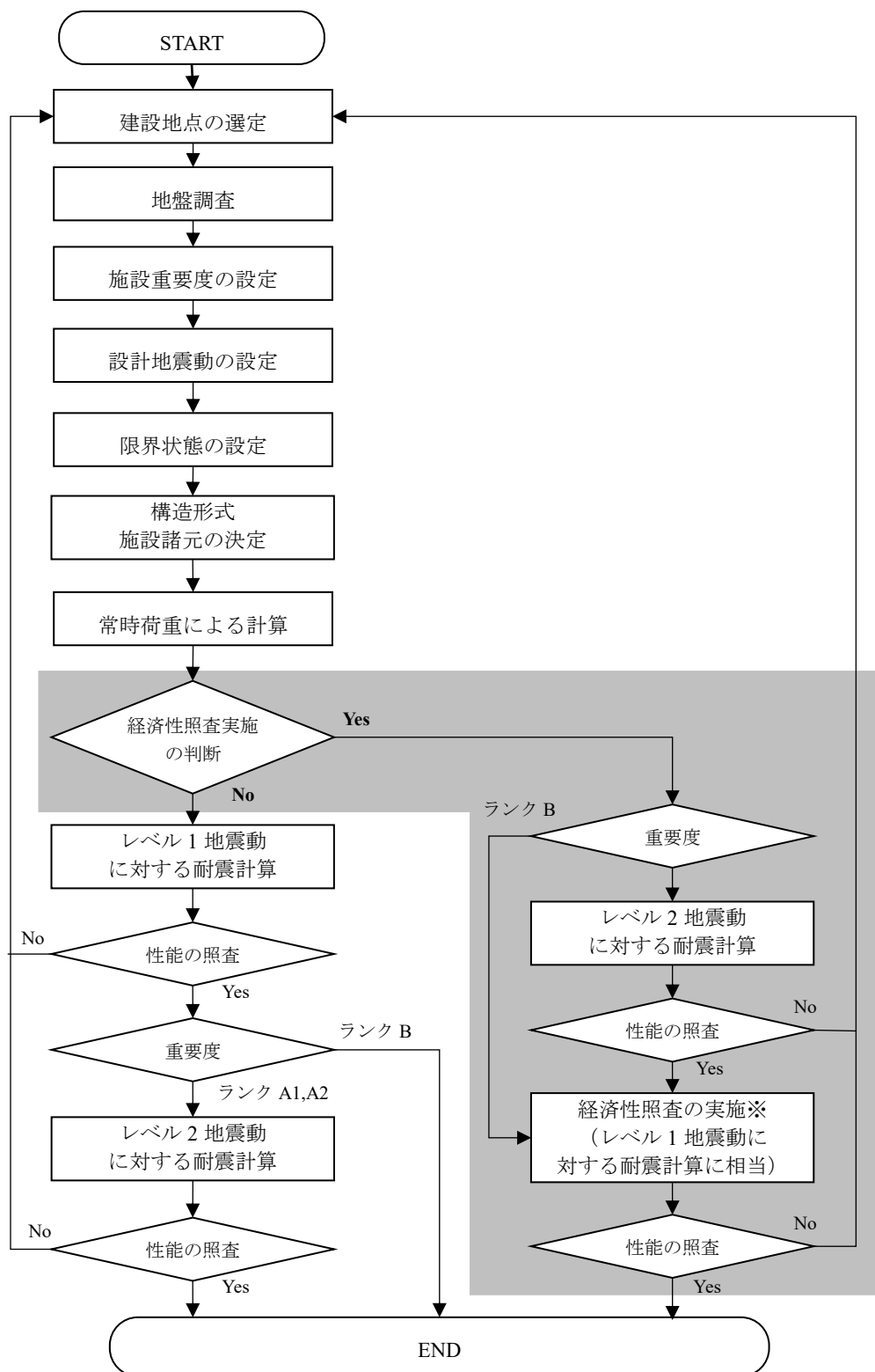
図 2.2 耐震設計のフロー（新設）
