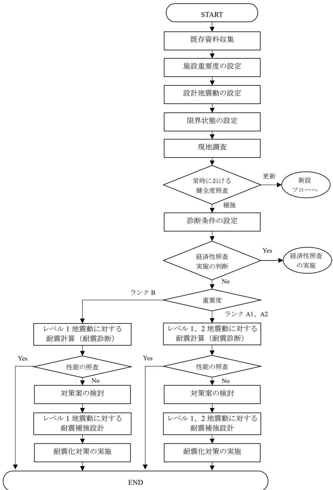
図 2.3 耐震設計のフロー（既設）
