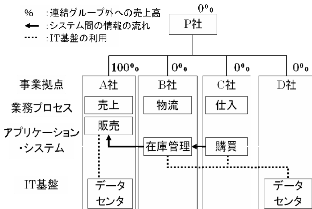
図表Ⅲ. 2－2 IT の評価範囲の例
