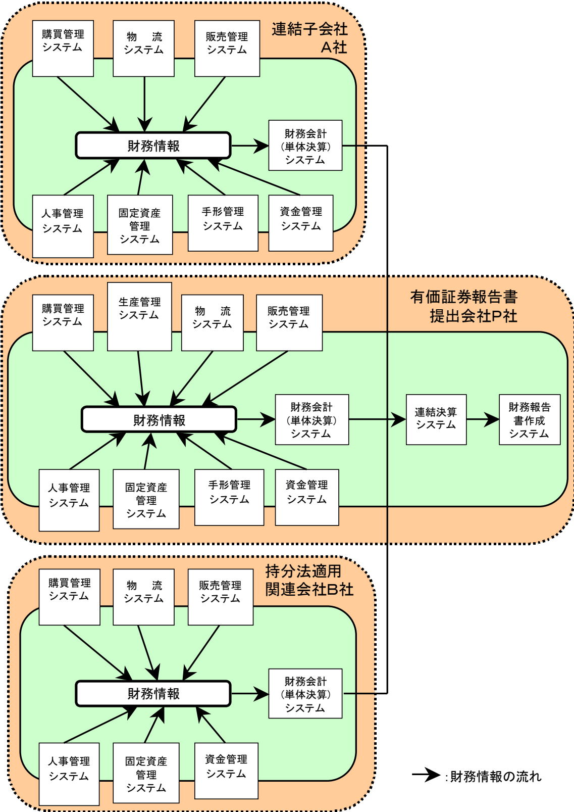
図表Ⅱ. 1－4 財務報告とアプリケーション・システムの関係
