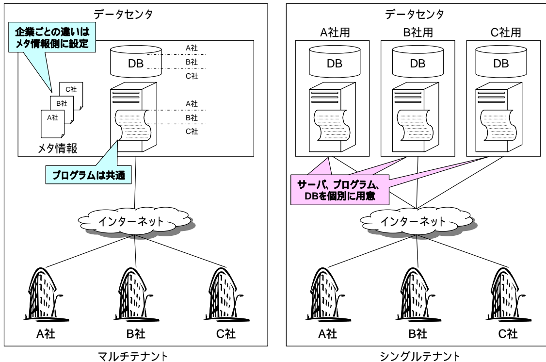
図 6 マルチテナントとシングルテナントの違い
