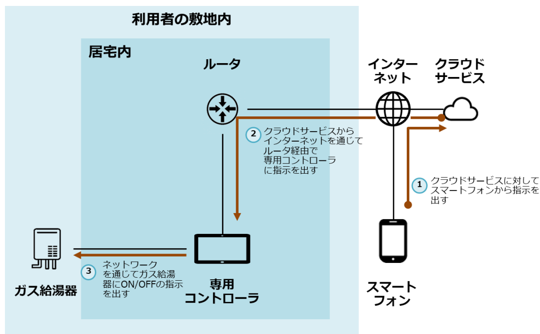
図 12 データフロー図(一部を抜粋)
