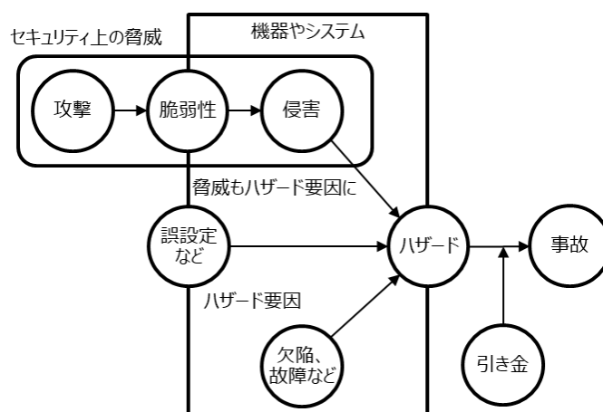
図6 セキュリティ上の問題がセーフティに影響を与えるモデル 14
