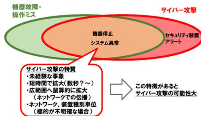
図 3-5 アラート発生要因の調査・整理
