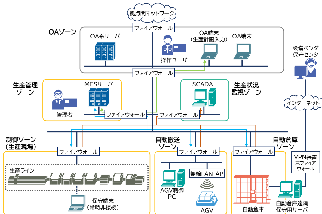
図 3-3 要件に対する各ゾーンでの対策(例)
