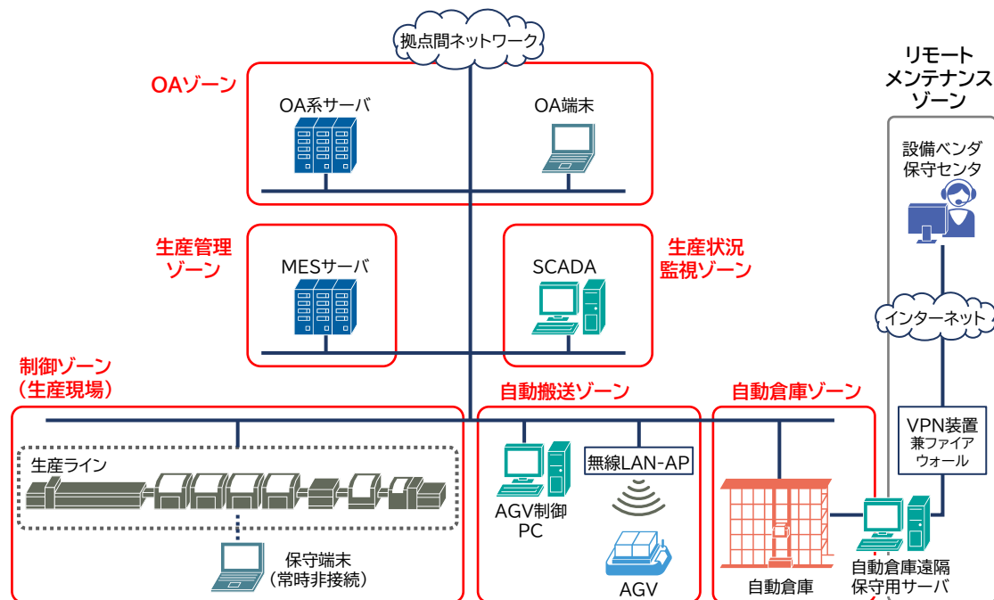
図 2-2 ゾーンの定義例
