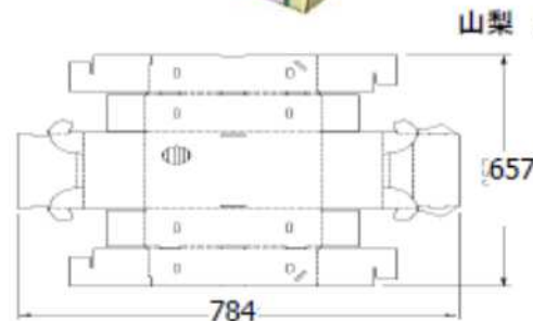
従来品 0.515 m 2 (100)
