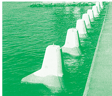
スラグ利用消波ブロックの敷設状況
