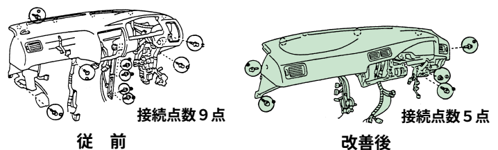
インパネの締結点数の減少
