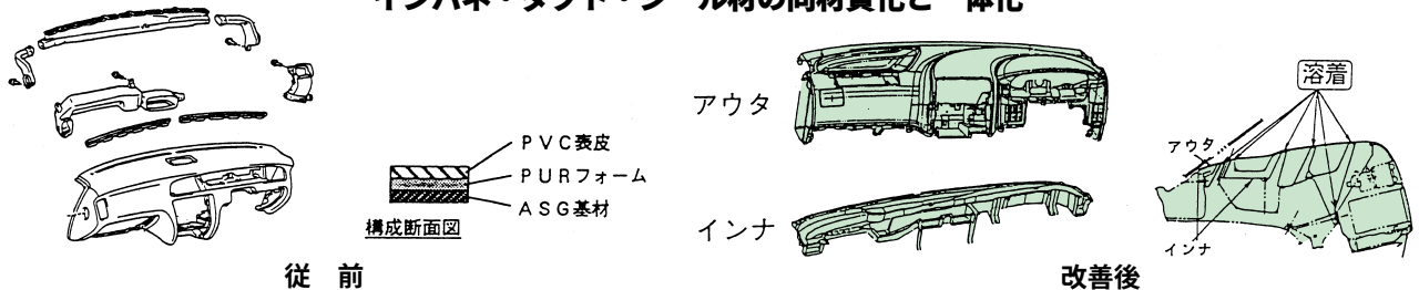
インパネ・ダクト・シール材の同材質化と一体化
