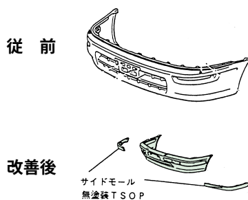
バンパーの損傷しやすい部分を別部品化
