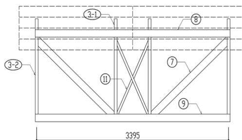
背面図
