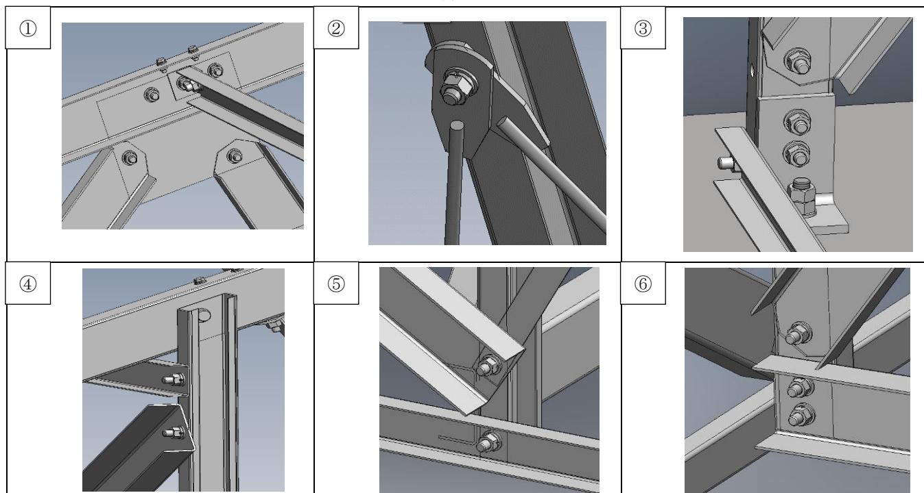
詳細図
