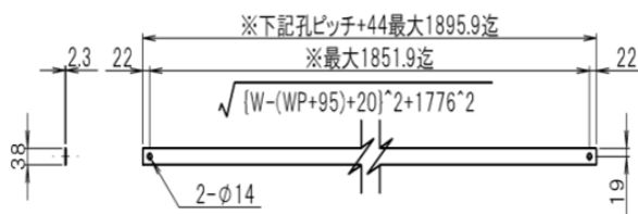
1 2 - 2 横材中央
