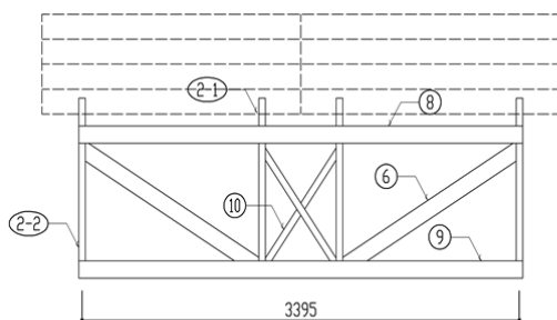
正面図
