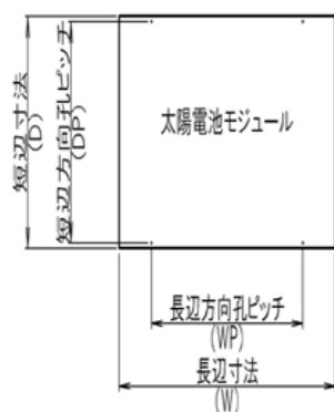
部品図 モジュール外形
