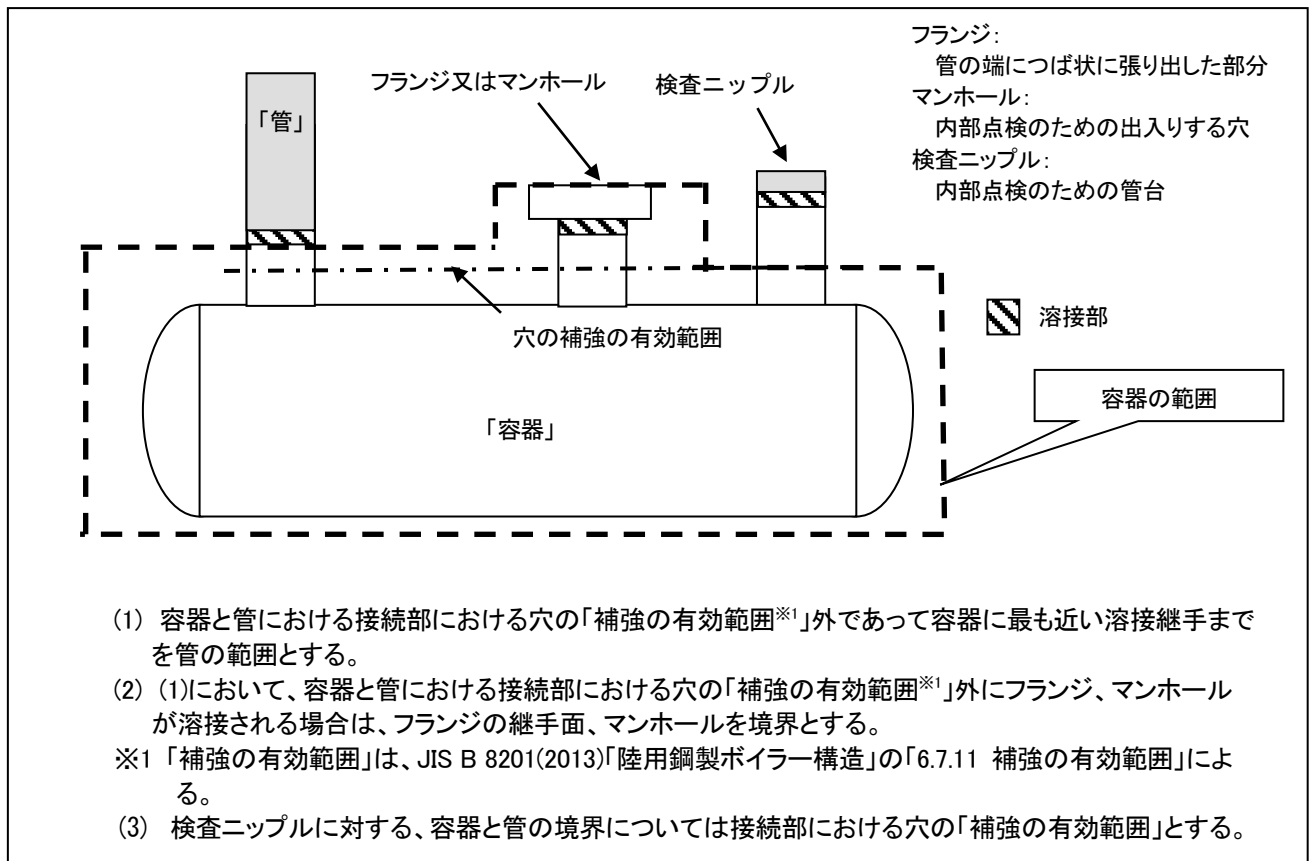
図2 容器と管の区分の例
