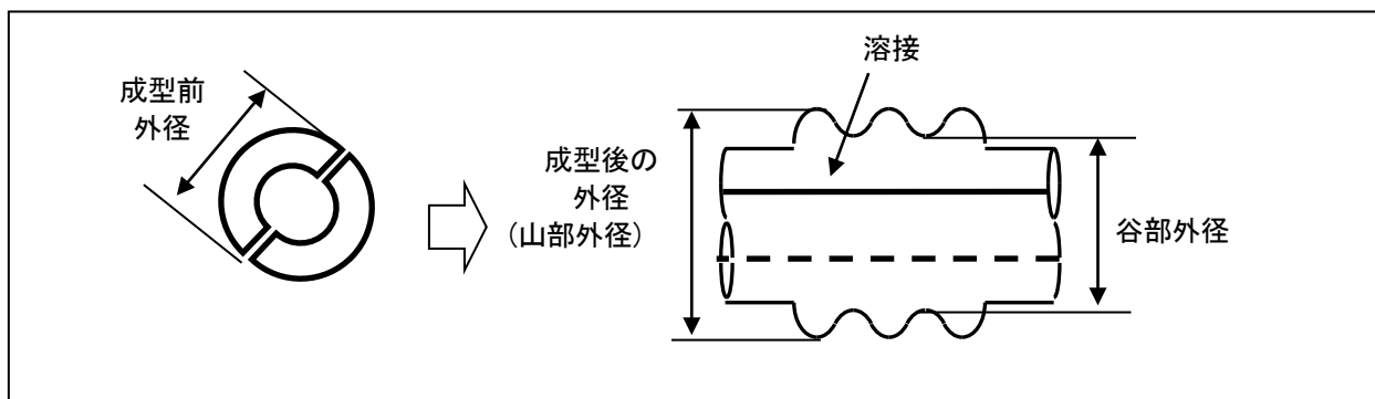
図4 ベローズの溶接事業者検査要否を決める外径寸法
