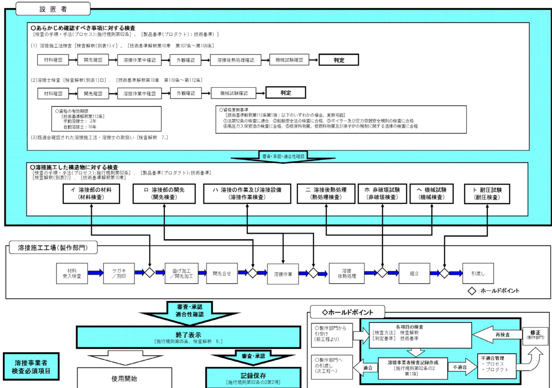
図 1 溶接事業者検査の実施に係るプロセスマップ
