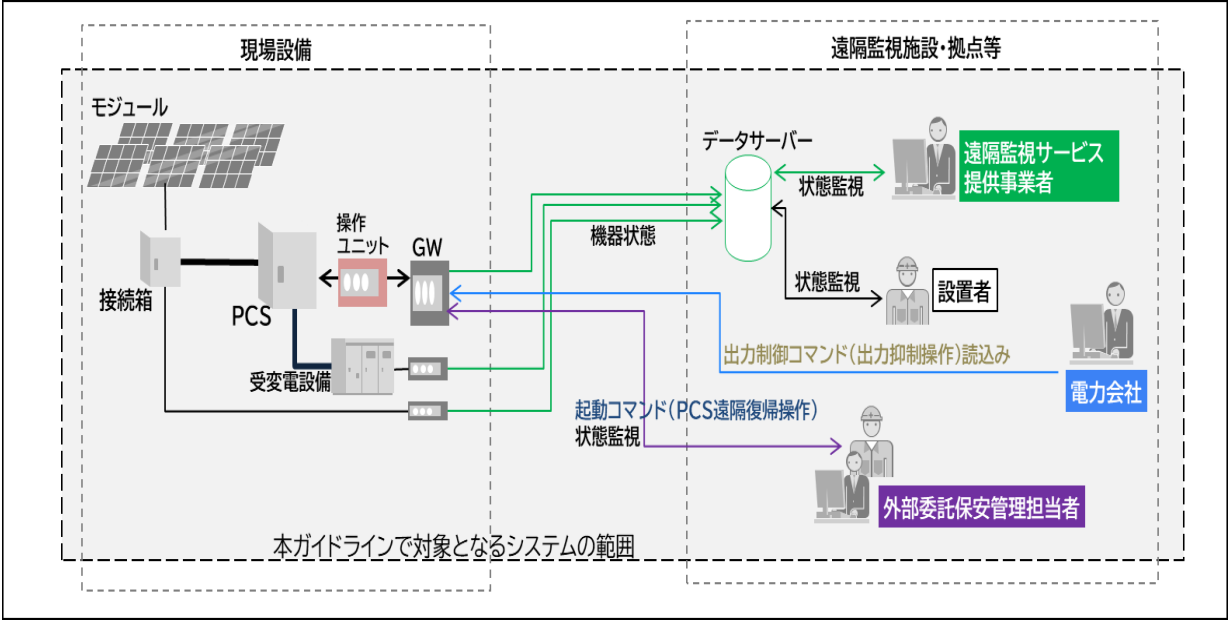
図2：発電設備の保安管理業務を外部委託する場合の対象システムの範囲の例（発電設備の出力制御コマンドが系統接続先の電力会社から別のシステムを介して伝達される例）
