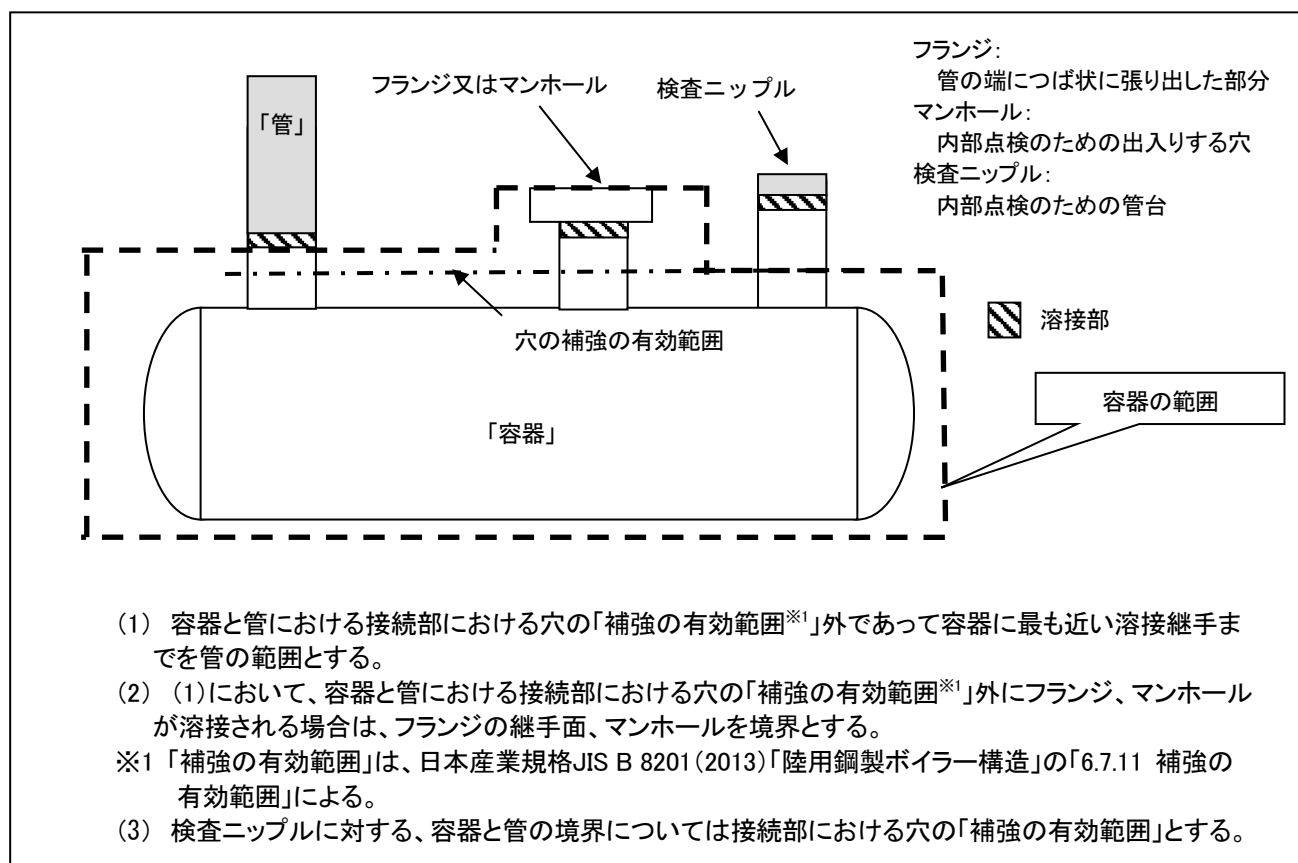
図2 容器と管の区分の例
