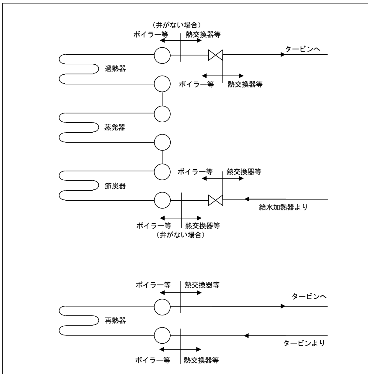
図 6 ボイラーと熱交換器等との境界
