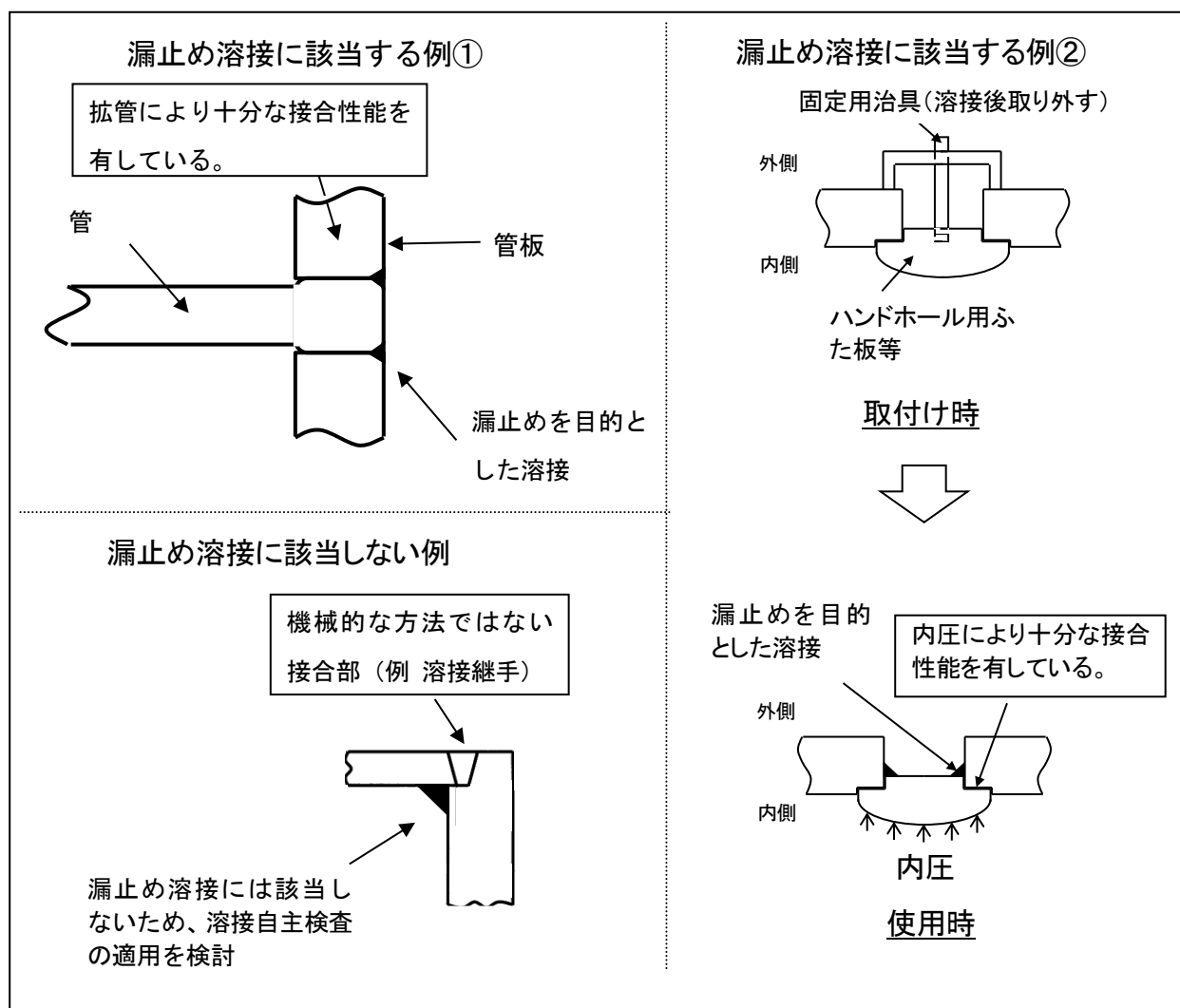
図 5 漏止め溶接に関する説明図
