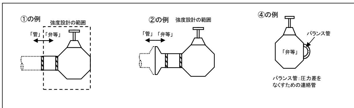
図3 「弁等」と「管」の境界の例示
