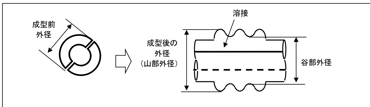
図4 ベローズの溶接自主検査要否を決める外径寸法
