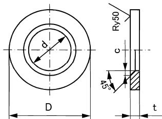
図 3 座金
