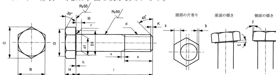
図 1 ボルト
