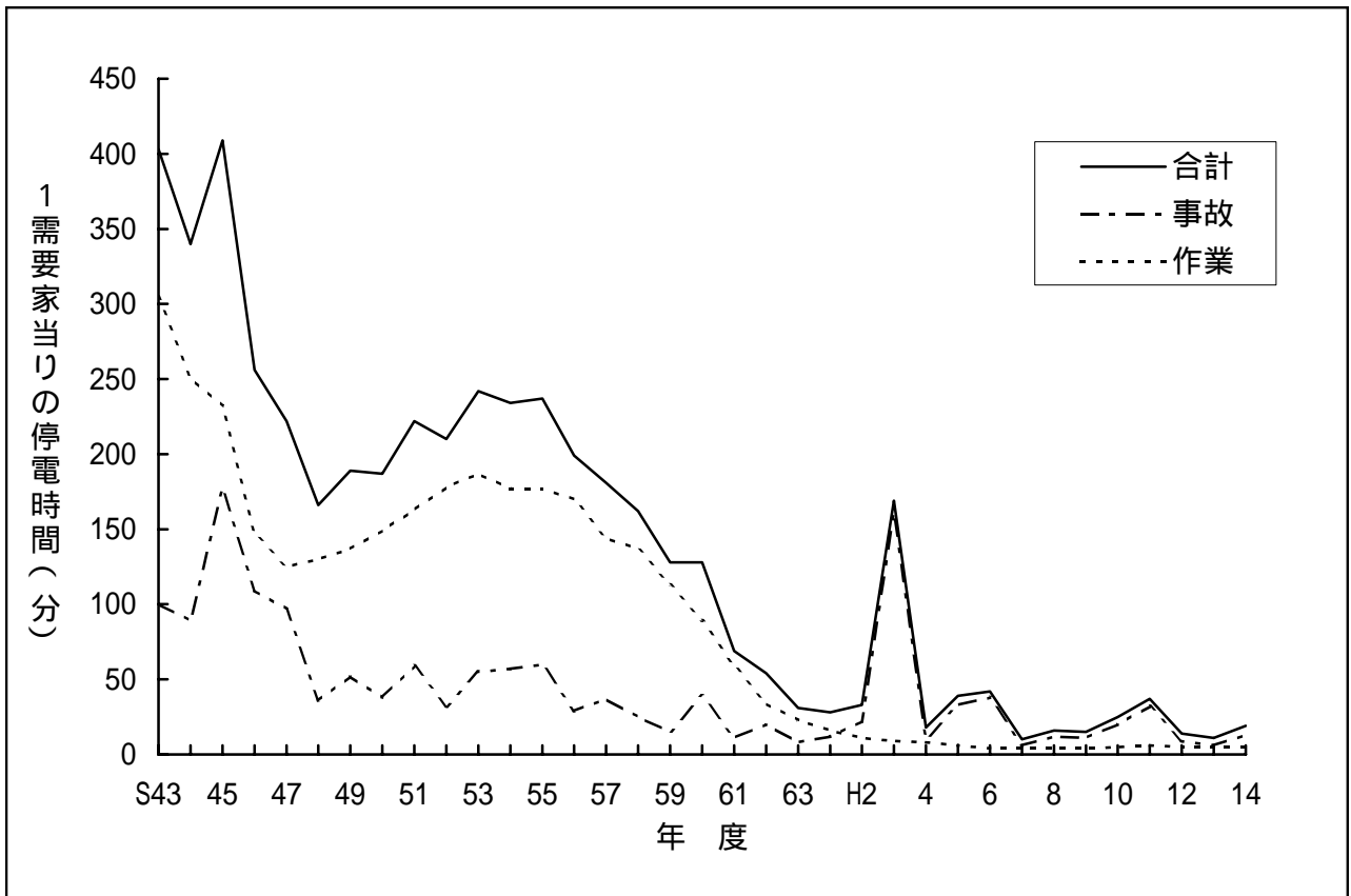
第1 - 2図 需要家停電時間の推移
