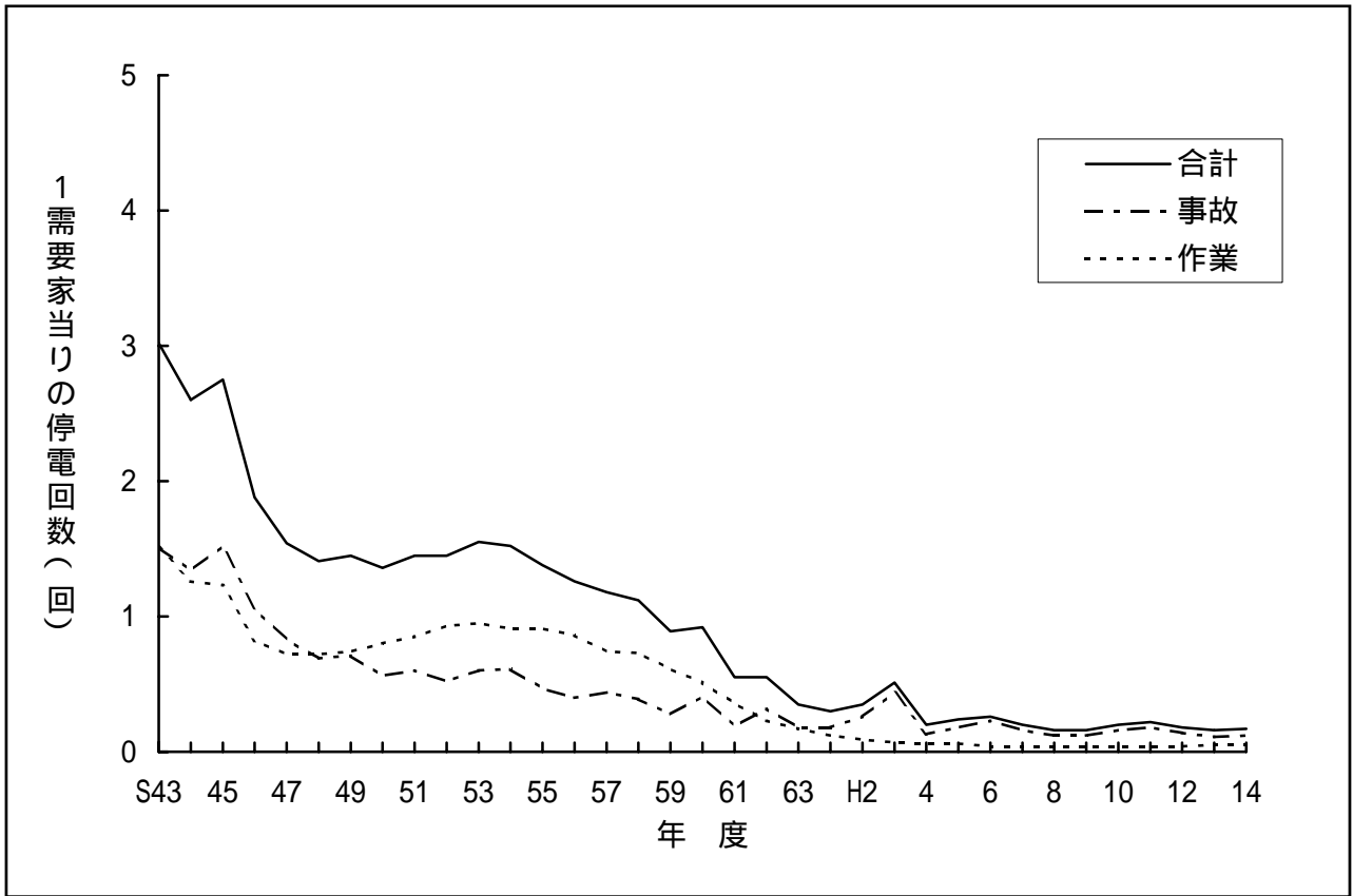
第1 - 1図 需要家停電回数の推移
