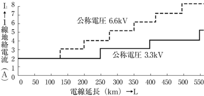
① 非接地式高压架空電線路の1線地絡電流
