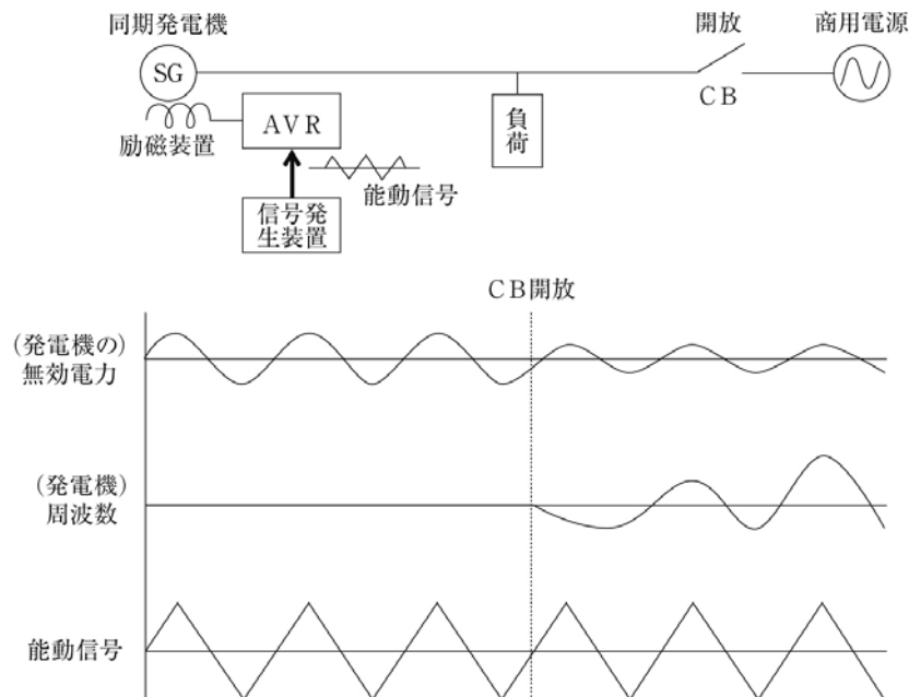
(b) 〈無効電力変動方式：同期発電機の例〉
