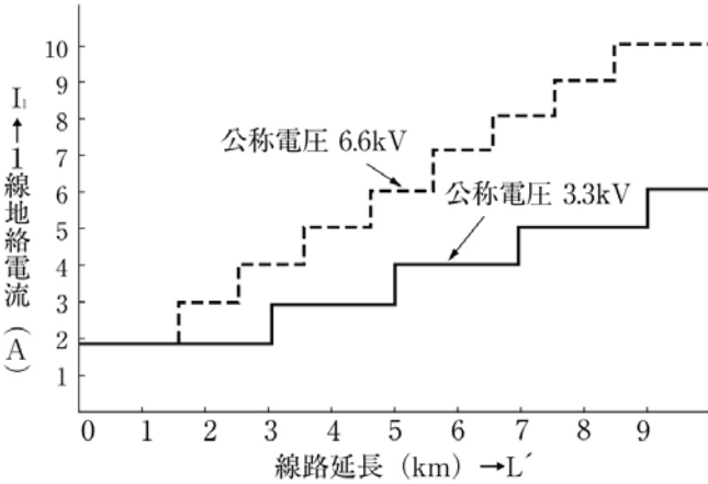
② 非接地式高压地中電線路の1線地絡電流
