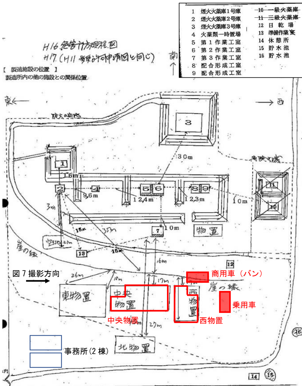
図1 工場配置図 (物的被害を赤字で記載)
