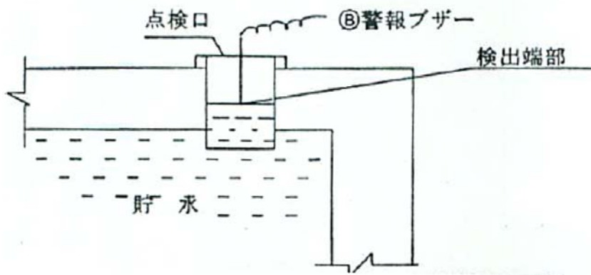
図－３ 点検口及び水位警報装置検出端部設置例
