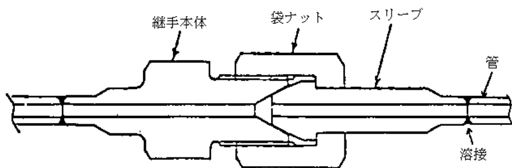
図4 小口径高圧用管継手型式
