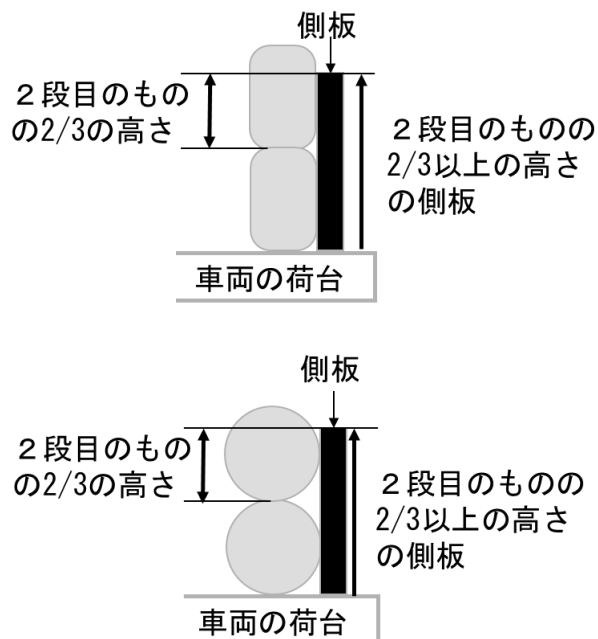
図 充填容器等を2段に積み重ねた場合の側板の高さ（概念図 上：縦積み、下：横積み）
