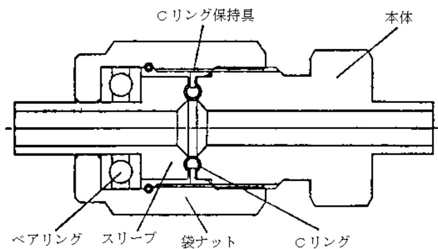
図4 小口径高圧用管継手型式
