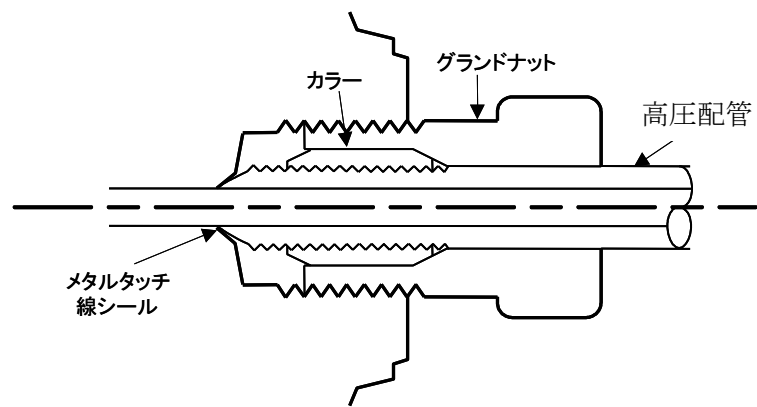
図6 コーン・スレッド型式
